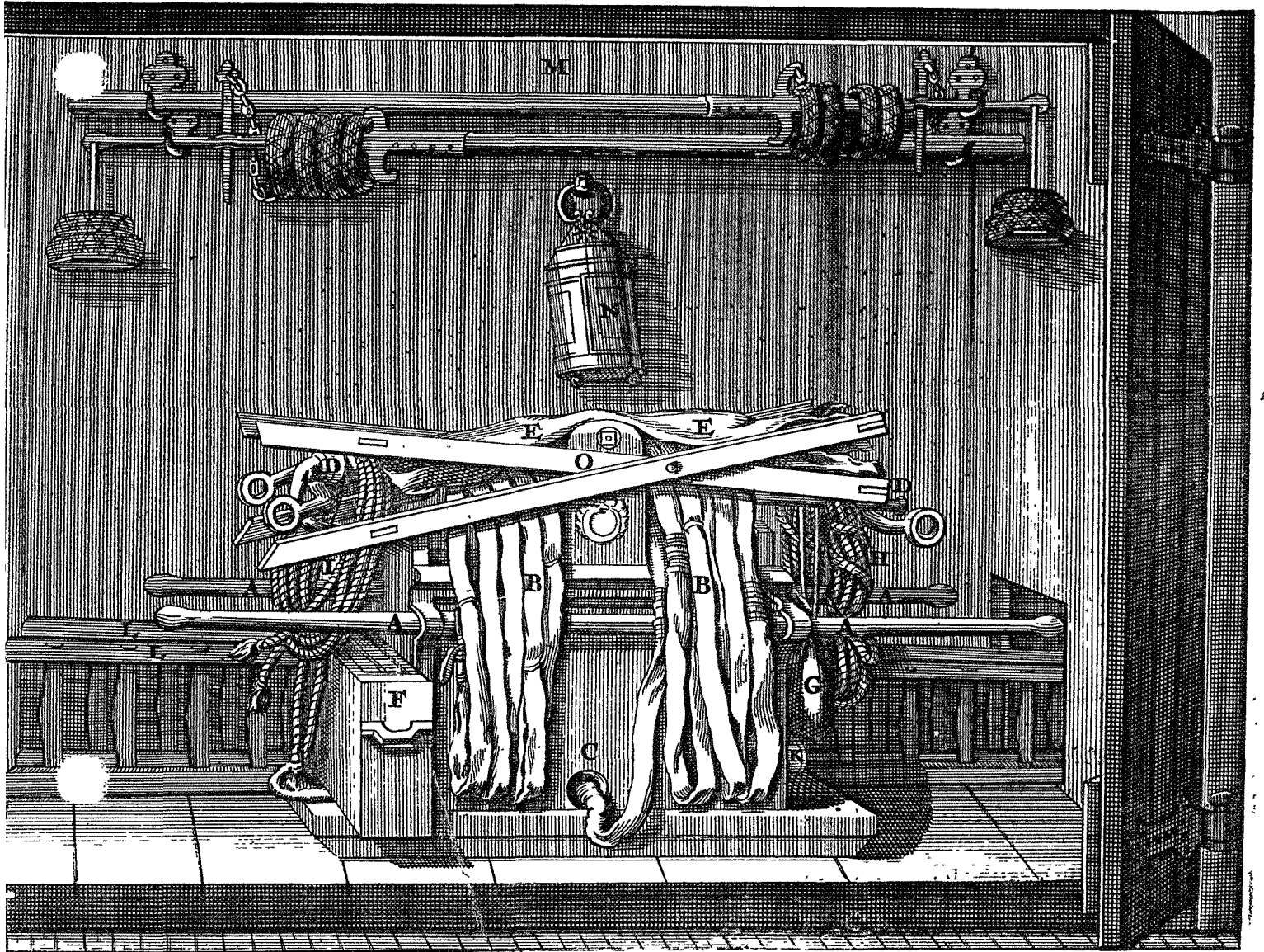
A HANDBOOMEN, steekende in de draag-beugels van de Spuit B. SPUIT-
